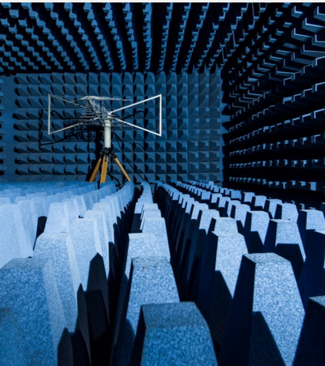
FULL ANECHOIC CHAMBRE 3 m x 3 m x 2,6 m
