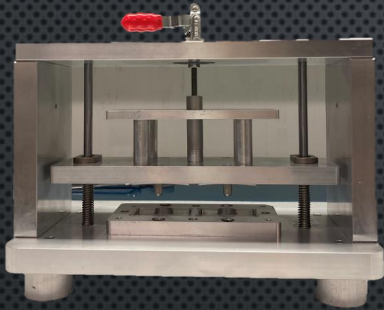
Press tool
