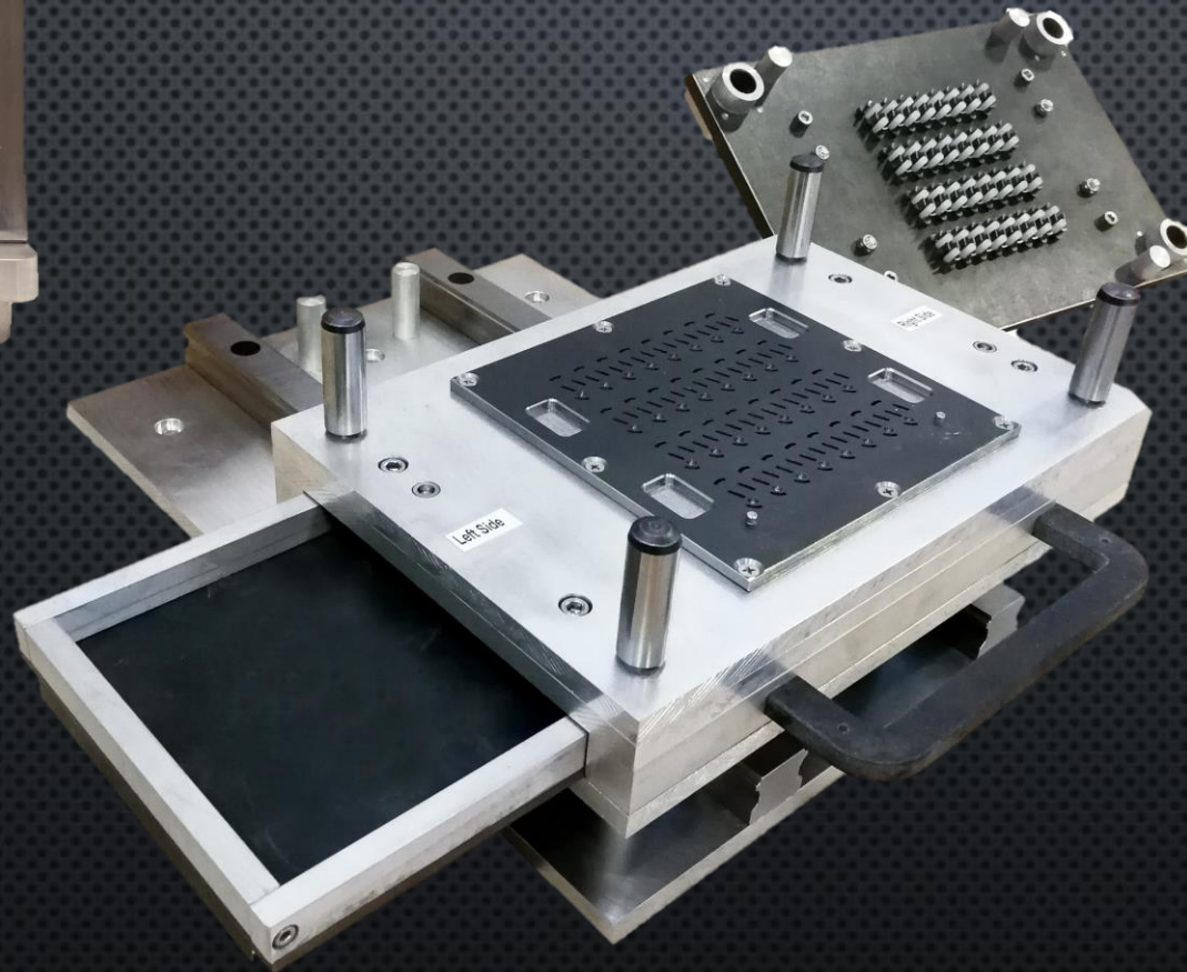
Depaneling press tool
